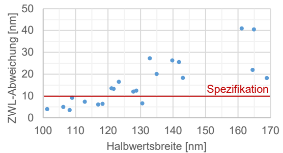
Abb. 17: Maximalabweichung in Abhängigkeit der HWB des FPI-Detektors
